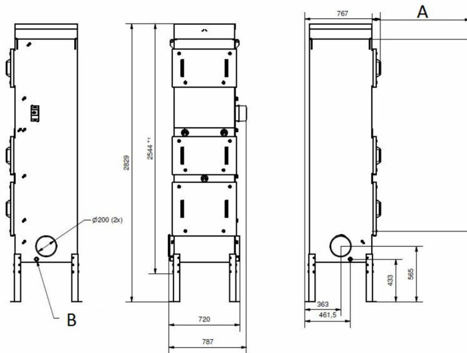
A) 1000 mm plads for filter service B) Drænstuds (x2)
